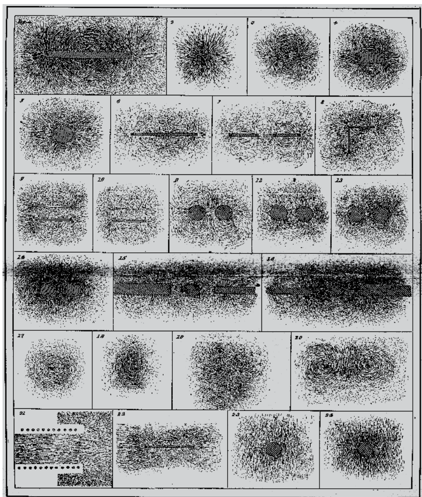
Abb. 10: Faraday: Magnetische Kraftlinien
