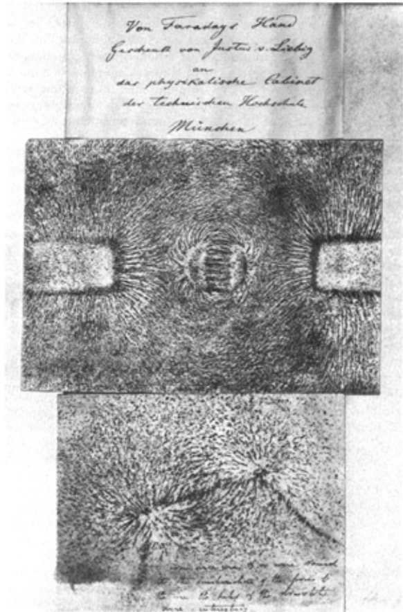
Abb. 11: Faraday: Kraftlinienbild. Von Faraday selbst 1850 mit Eisenspänen erzeugt und fixiert.
