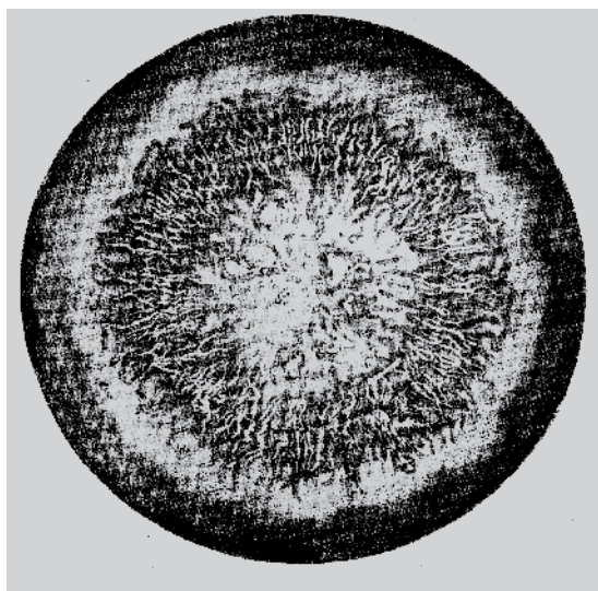
Abb. 4 - 7: Lichtenberg-Figuren
