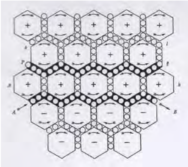
Abb. 12: Maxwell: Äthermodell
