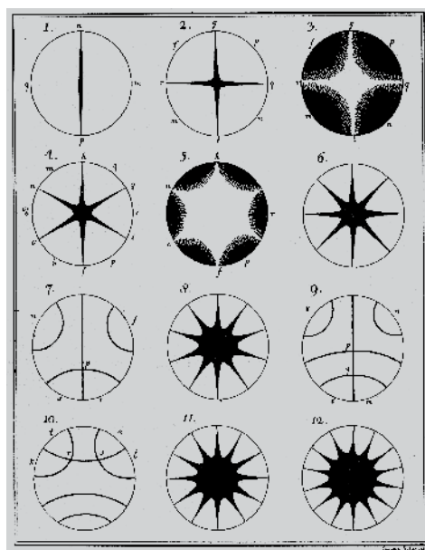
Abb. 9: Chladni: Klangfiguren
