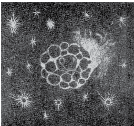
Abb.2: Lichtenberg-Figur
